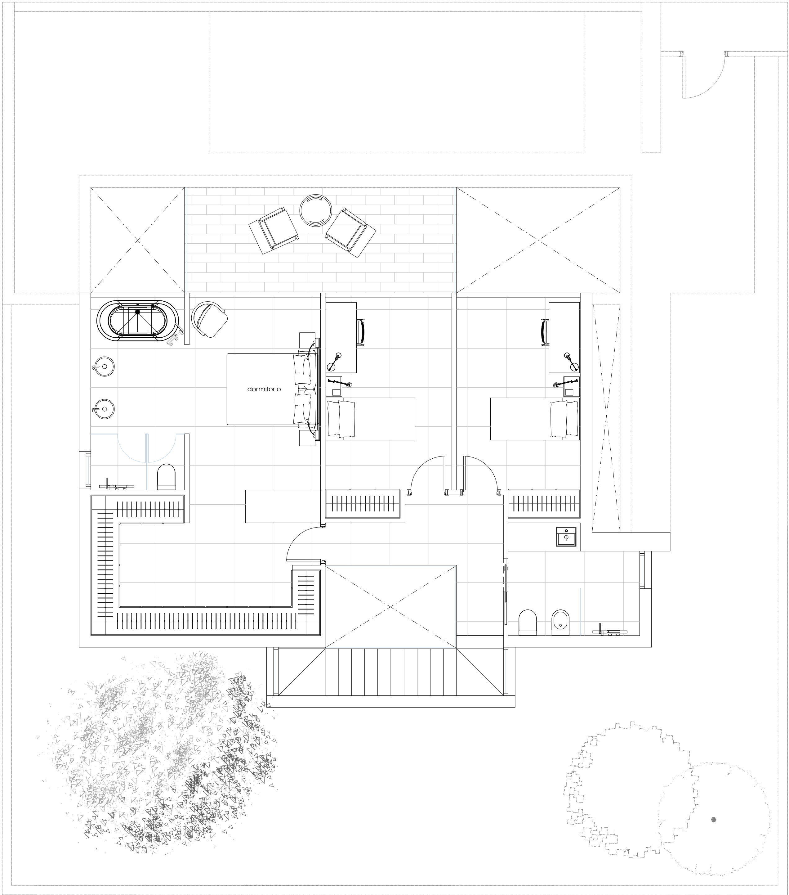
planta primera
