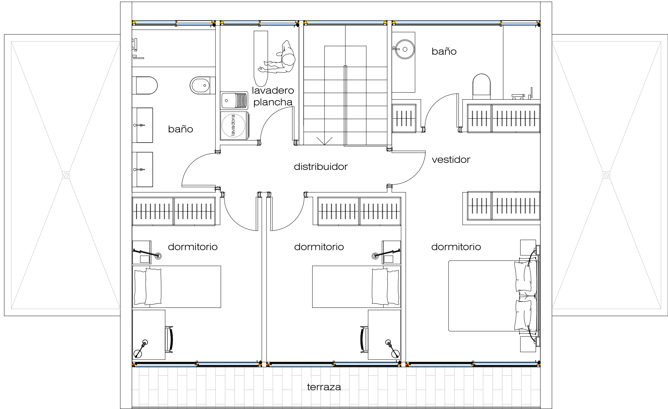
planta primera
