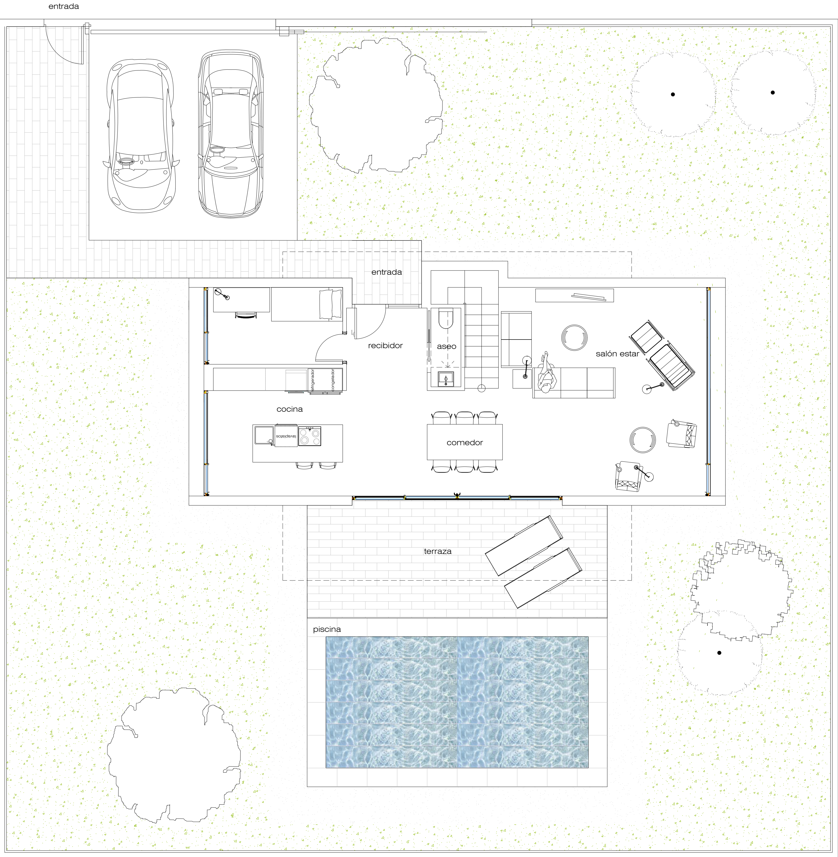
planta baja
