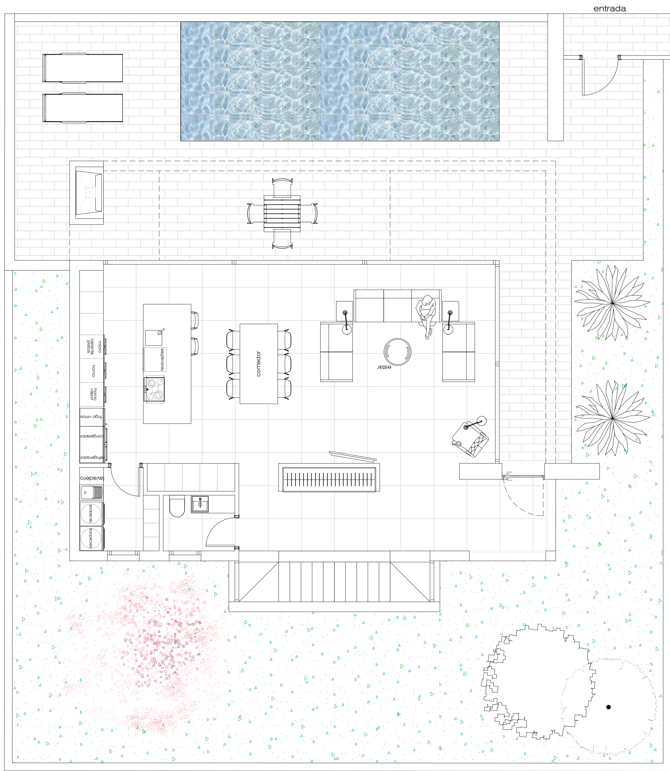
planta baja
